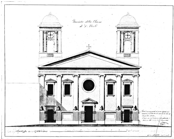
Fig. 1. Progetto originale della chiesa di S. Nicolò dei Greci in Trieste.
